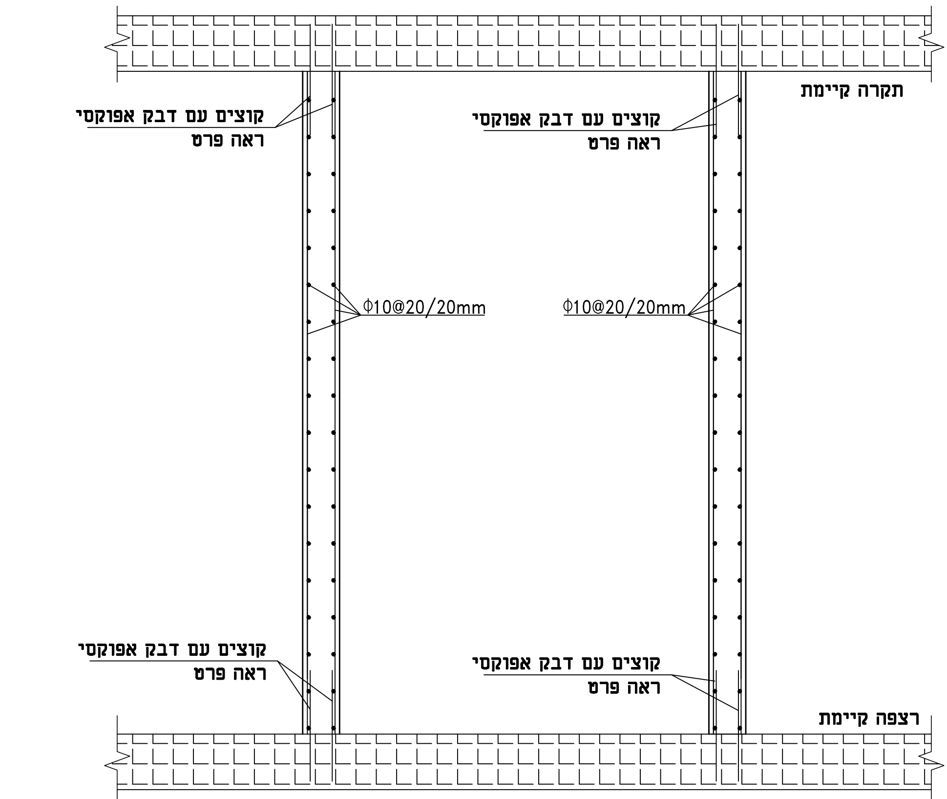
פרט קיר בטון מגו למח"מ 1:20
